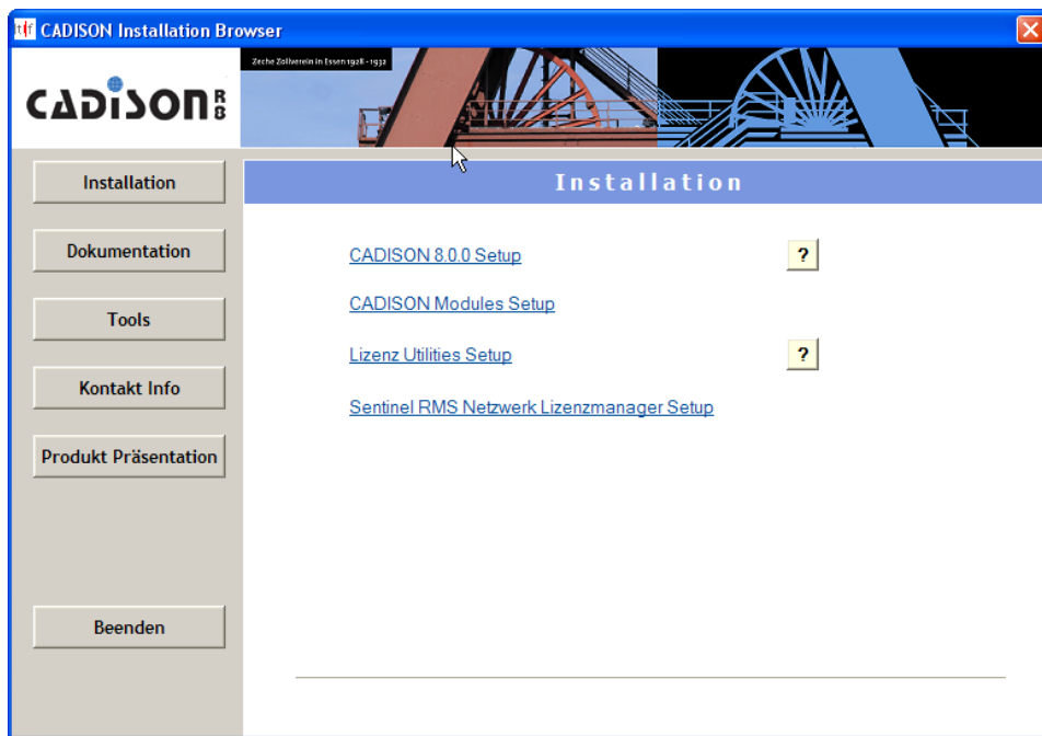
Abbildung 3: CADISON Installationsbrowser
